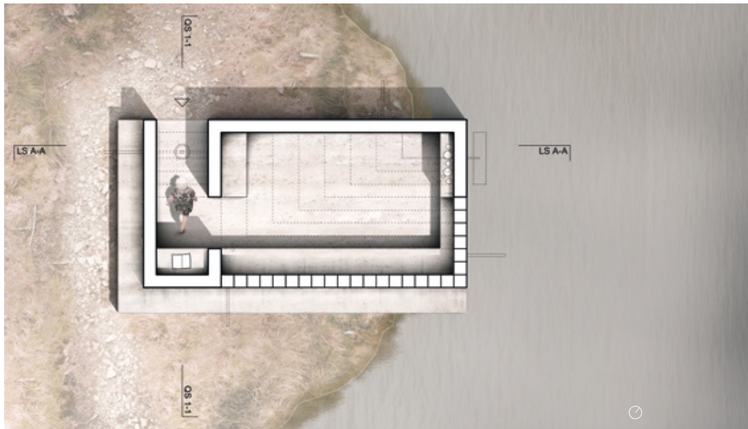
Grundriss
