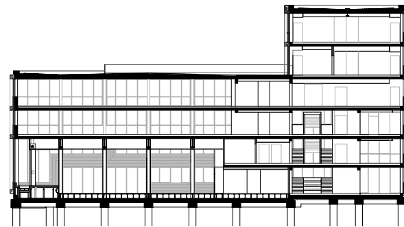
Längsschnitt
